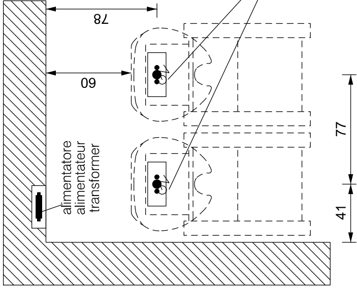
POSIZIONE DEL CENTRO SCARICO ENCOMBREMENT TOTAL SITUATION OF THE DRAINING CENTER
