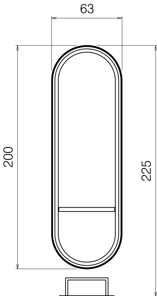
VISTA FRONTALE
