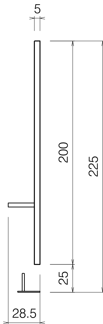
VISTA LATERALE
