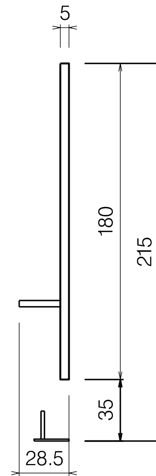
VISTA LATERALE
