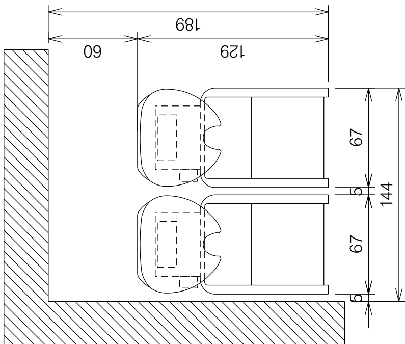
INGOMBRO TOTALE ENCOMBREMENT TOTAL TOTAL ENCUMBRANCE
