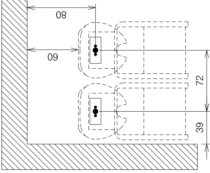
POSIZIONE DEL CENTRO SCARICO POSITION DU CENTRE DE L'ECOULEMENT SITUATION OF THE DRAINING CENTER
